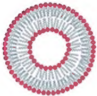
liposome
